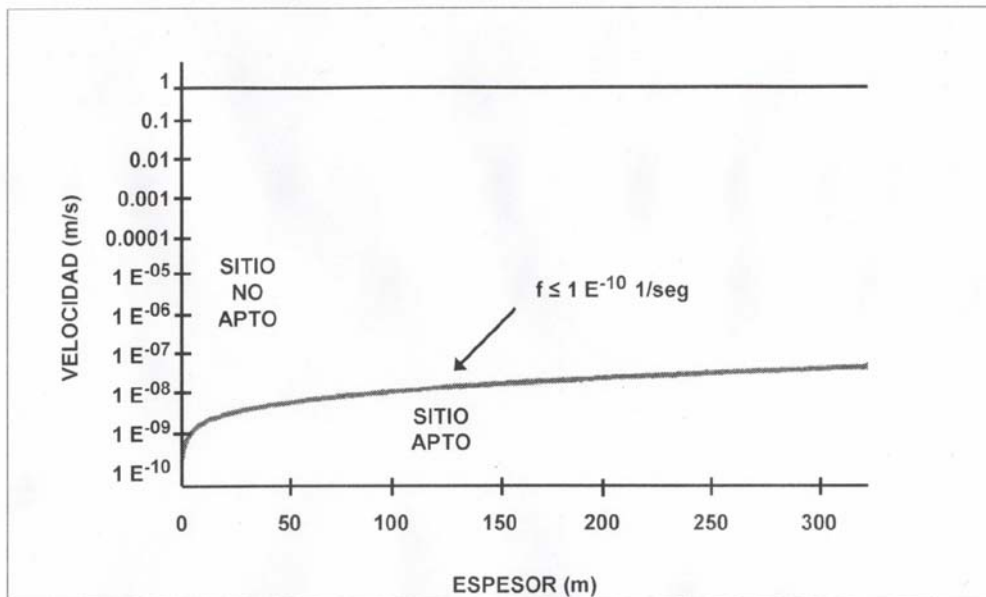
Gráfica 1. Tránsito de infiltración aceptable para los sitios de confinamiento de residuos peliarosos
