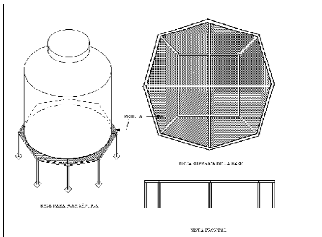
FIGURA 5. BASE PARA FOSA SEPTICA VERTICAL (figura ilustrativa)
