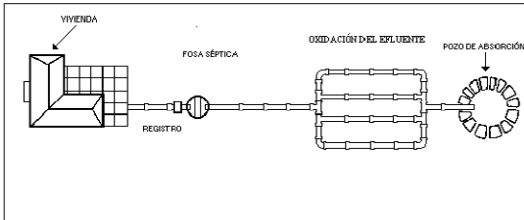
FIGURA 1. SISTEMA DE TRATAMIENTO FOSA SEPTICA (figura ilustrativa)
