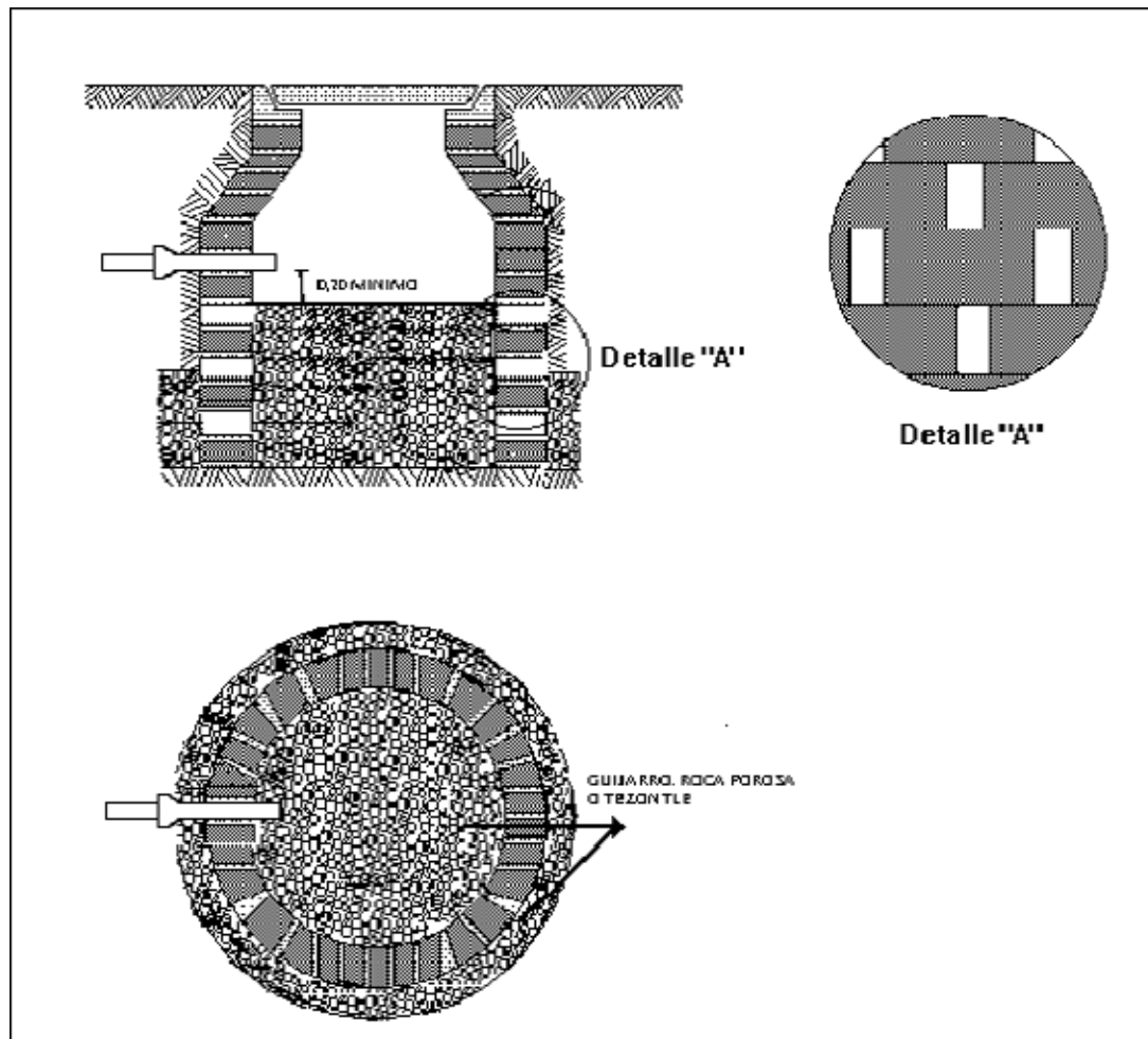
FIGURA 9. POZO DE ABSORCION (figura ilustrativa)
