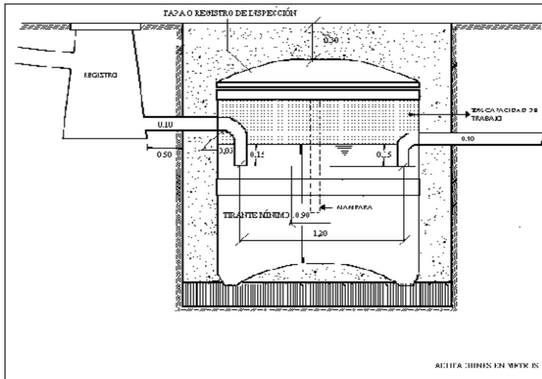
FIGURA 2. FOSA SEPTICA PREFABRICADA (figura ilustrativa)
