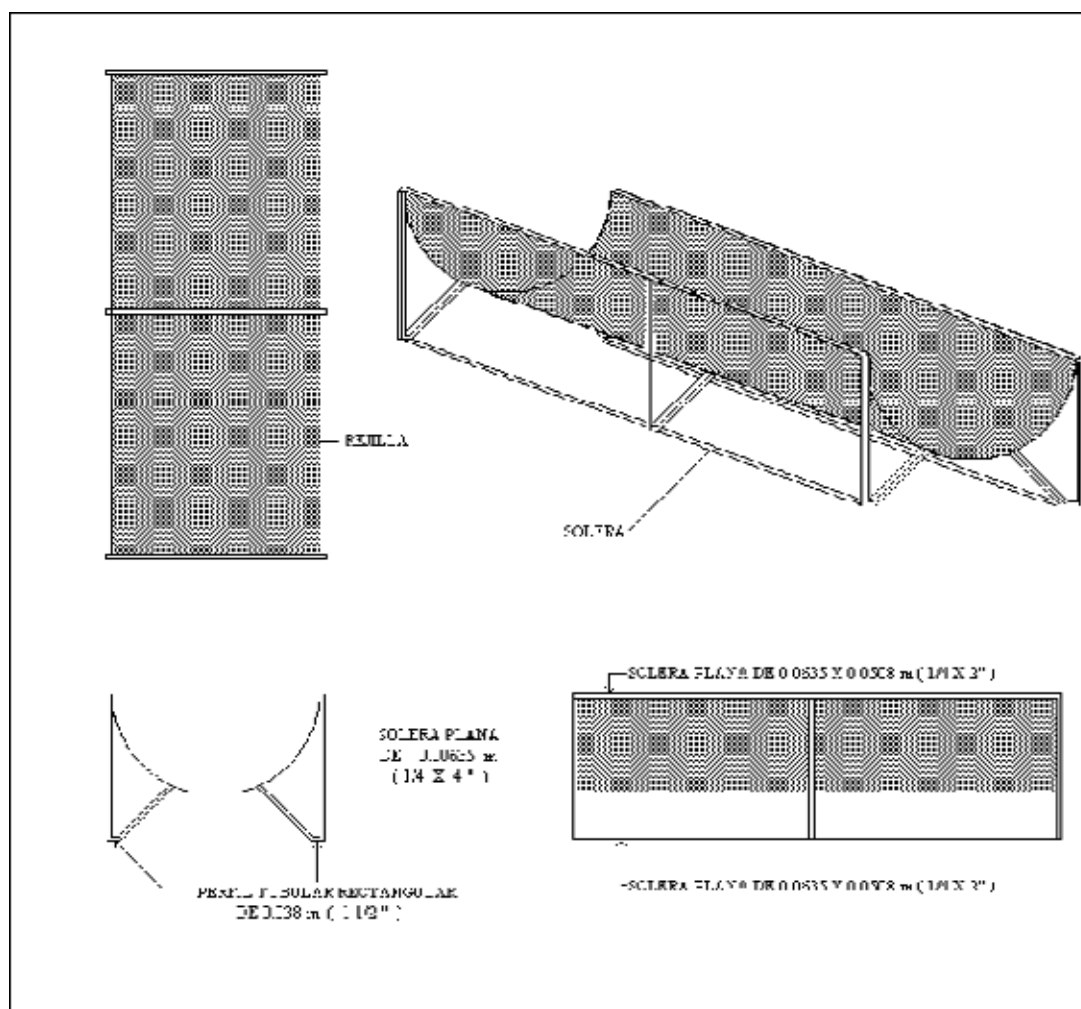
FIGURA 6. BASE PARA FOSA SEPTICA HORIZONTAL (figura ilustrativa)
