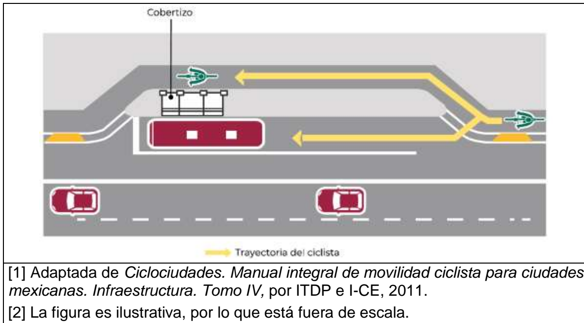
Figura 63.- Parada de transporte público con desvío ciclista y bahía [1] [2]
