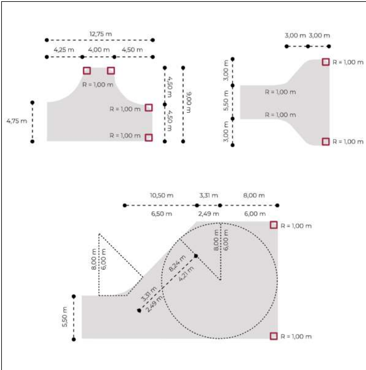
Figura 97.- Tipos de retorno para barreras de borde [1] [2]
