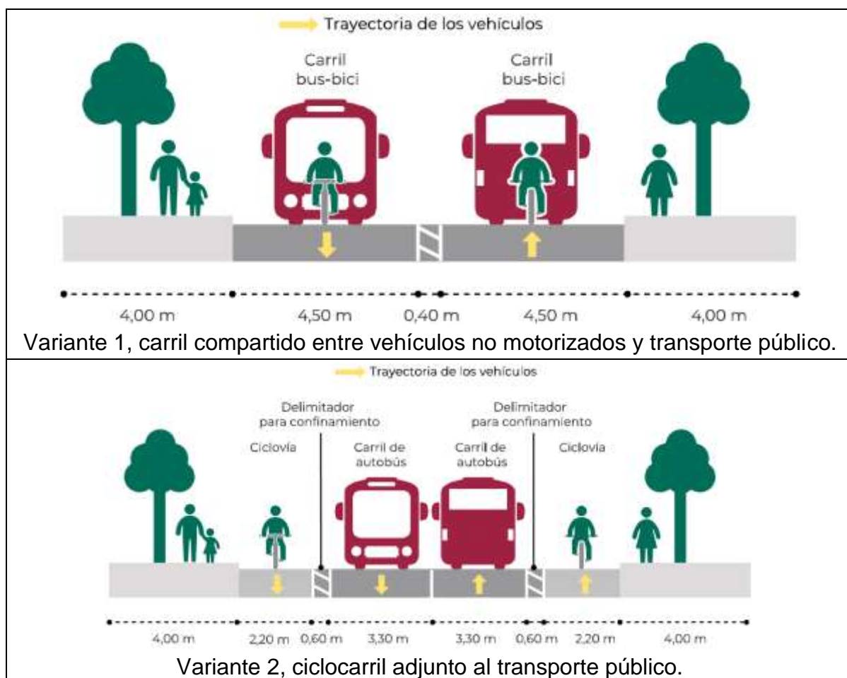
Figura 60.- Perfiles tipo de vías ciclistas compartidas con transporte público [1] [2] [3]
