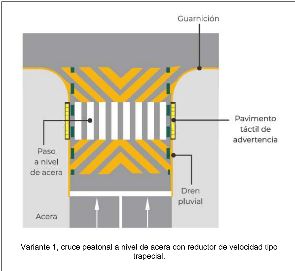
Figura 45.- Cruce peatonal a nivel de acera (planta) [1] [2] [3]
