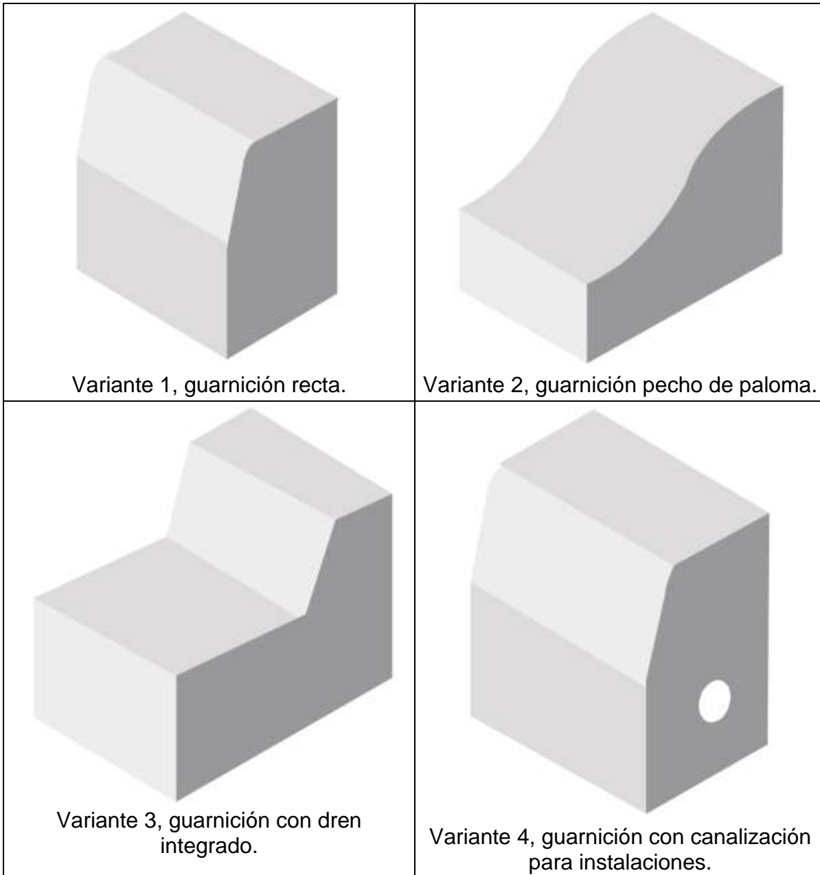
Figura 32.- Tipos de guarniciones [1] [2]
