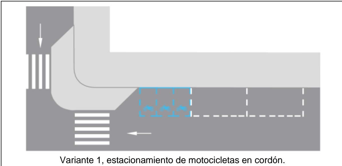
Figura 74.- Disposición de los cajones de motocicletas en relación con la franja de estacionamiento general [1] [2]
