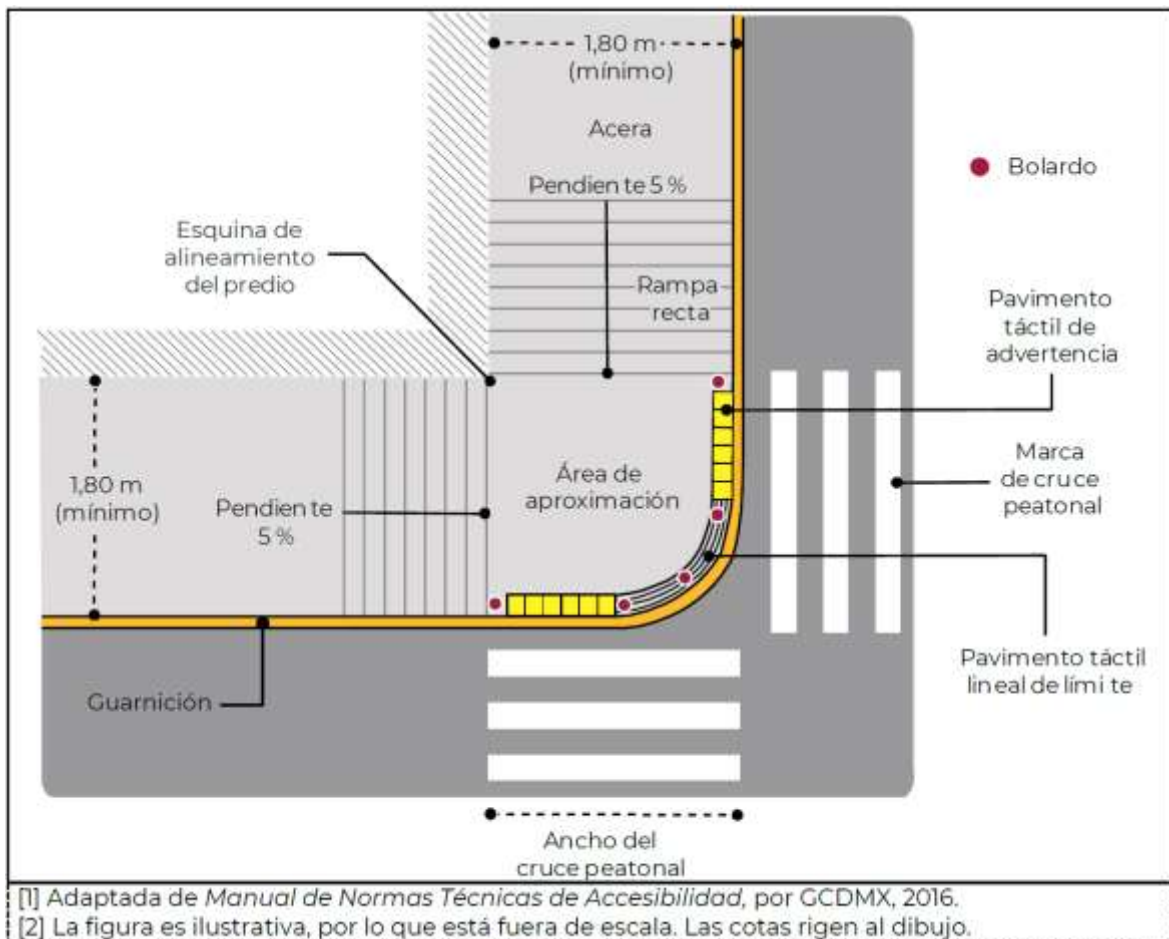
Figura 33.- Rampa con abanico (planta) [1] [2]
