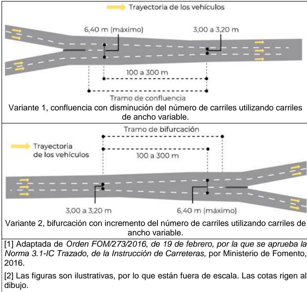
Figura 26.- Modificación de número de carriles con ancho variable [1] [2]
