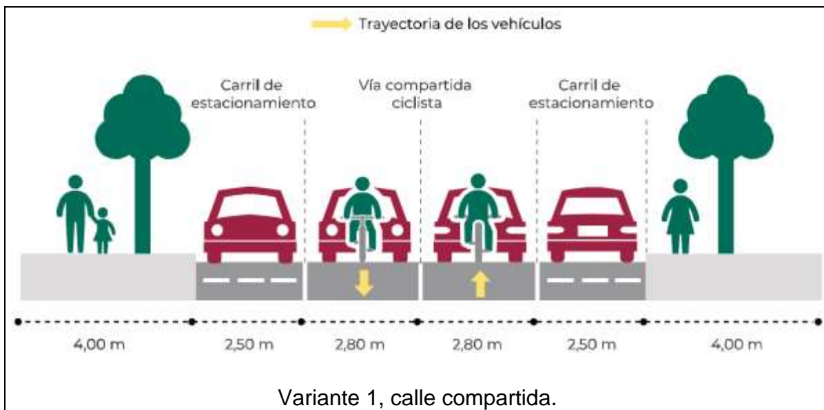
Figura 48.- Perfil tipo de vía ciclista con prioridad de uso [1] [2] [3]
