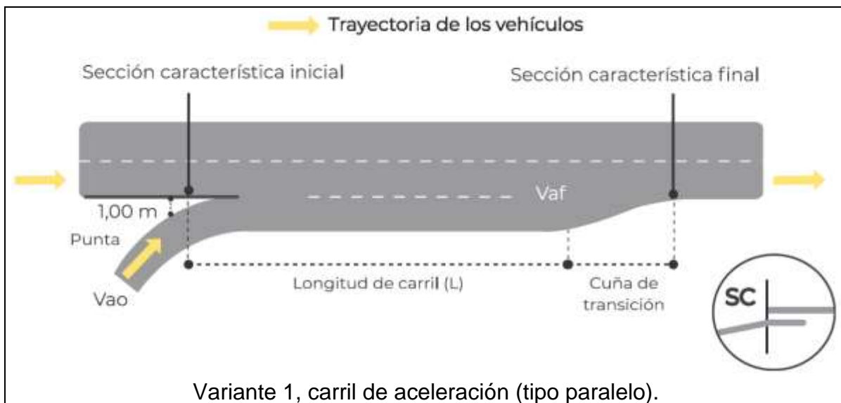
Figura 22.- Carriles de cambio de velocidad [1] [2] [a] [b]
