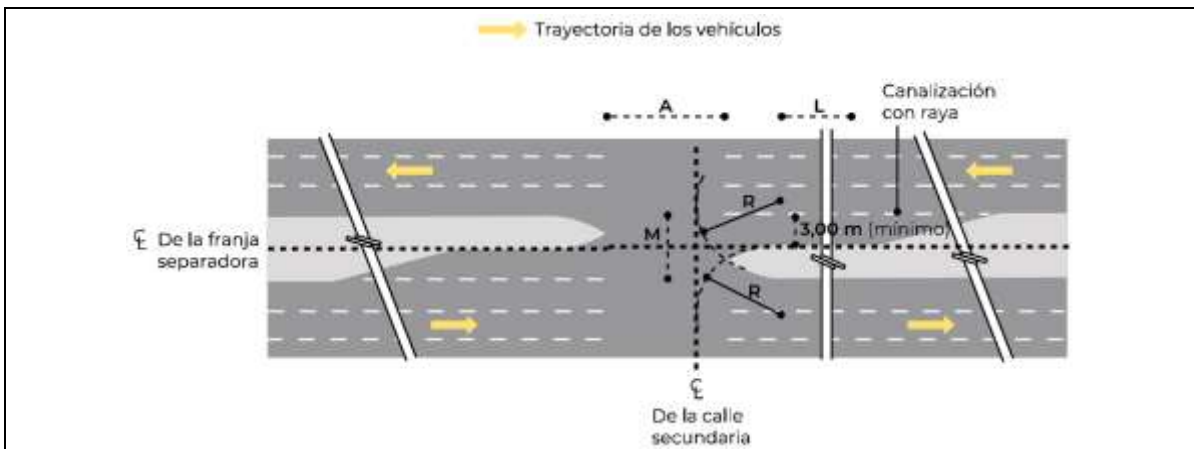
Figura 84.- Diseños de carril en la faja separadora central con remate en forma de punta de bala [1] [2]
