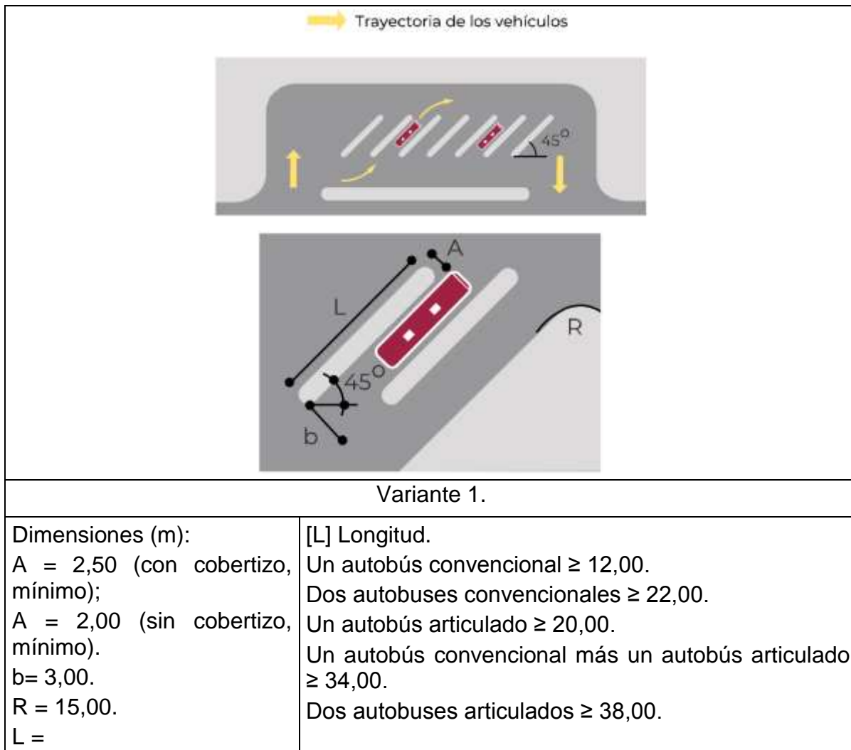
Figura 81.- Paraderos para el transporte público de pasajeros [1] [2]
