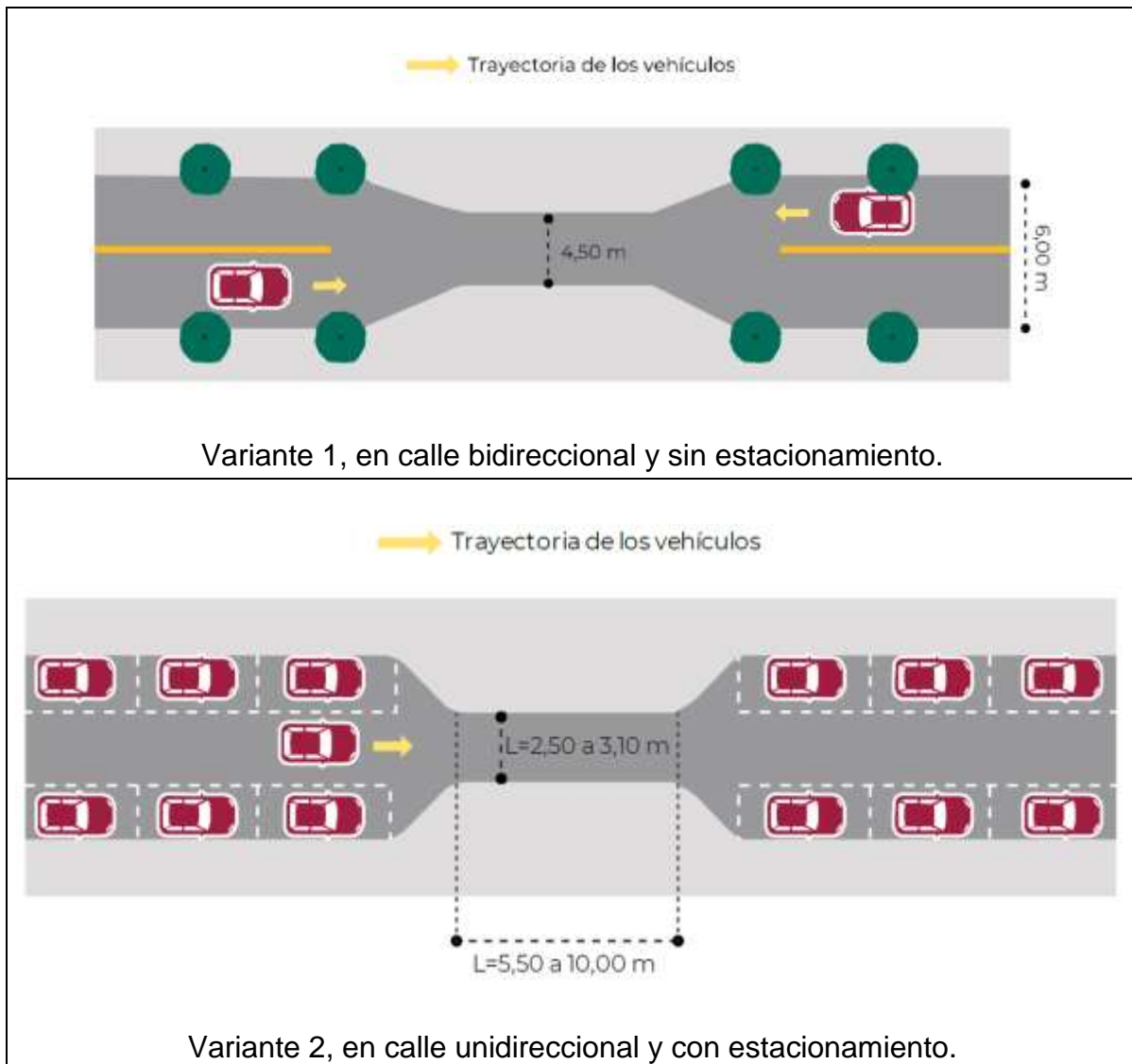
Figura 106.- Tipos de estrechamientos laterales [1] [2]
