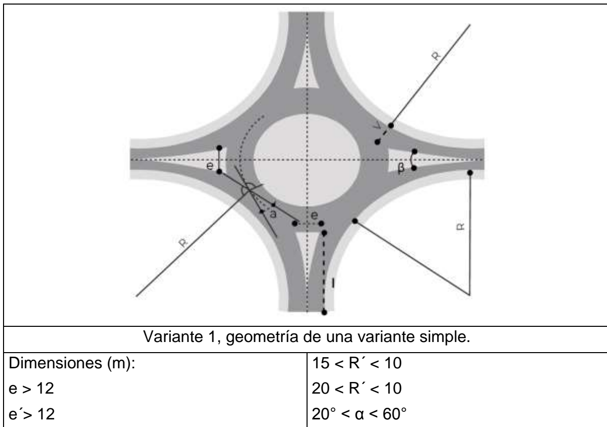
Figura 90.- Configuraciones de la glorieta simple. [1] [2]
