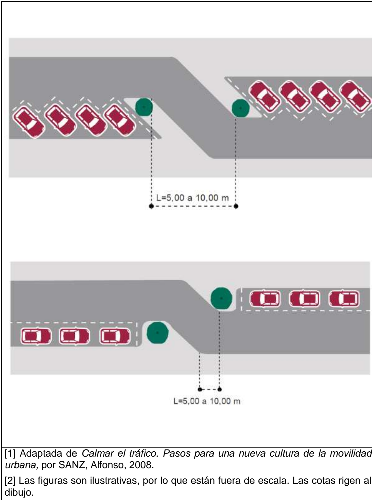
Figura 102.- Zigzag creados por estacionamiento alternado [1] [2]
