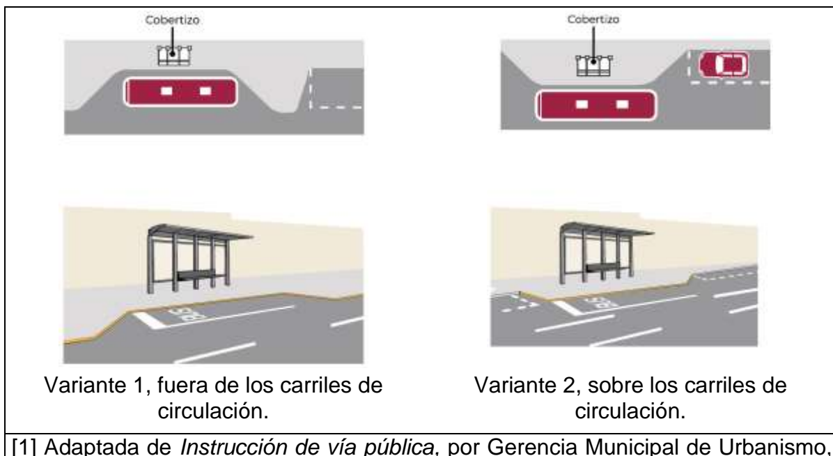
Figura 77.- Tipos de paradas de transporte público [1] [2]
