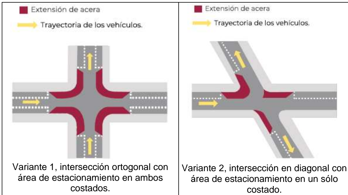
Figura 38.- Extensiones de acera [1] [2]
