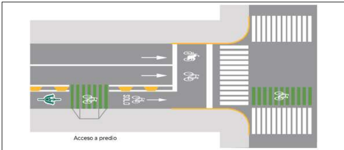
Figura 51.- Disposición del delimitador para confinamiento en ciclovías unidireccionales [1] [2]
