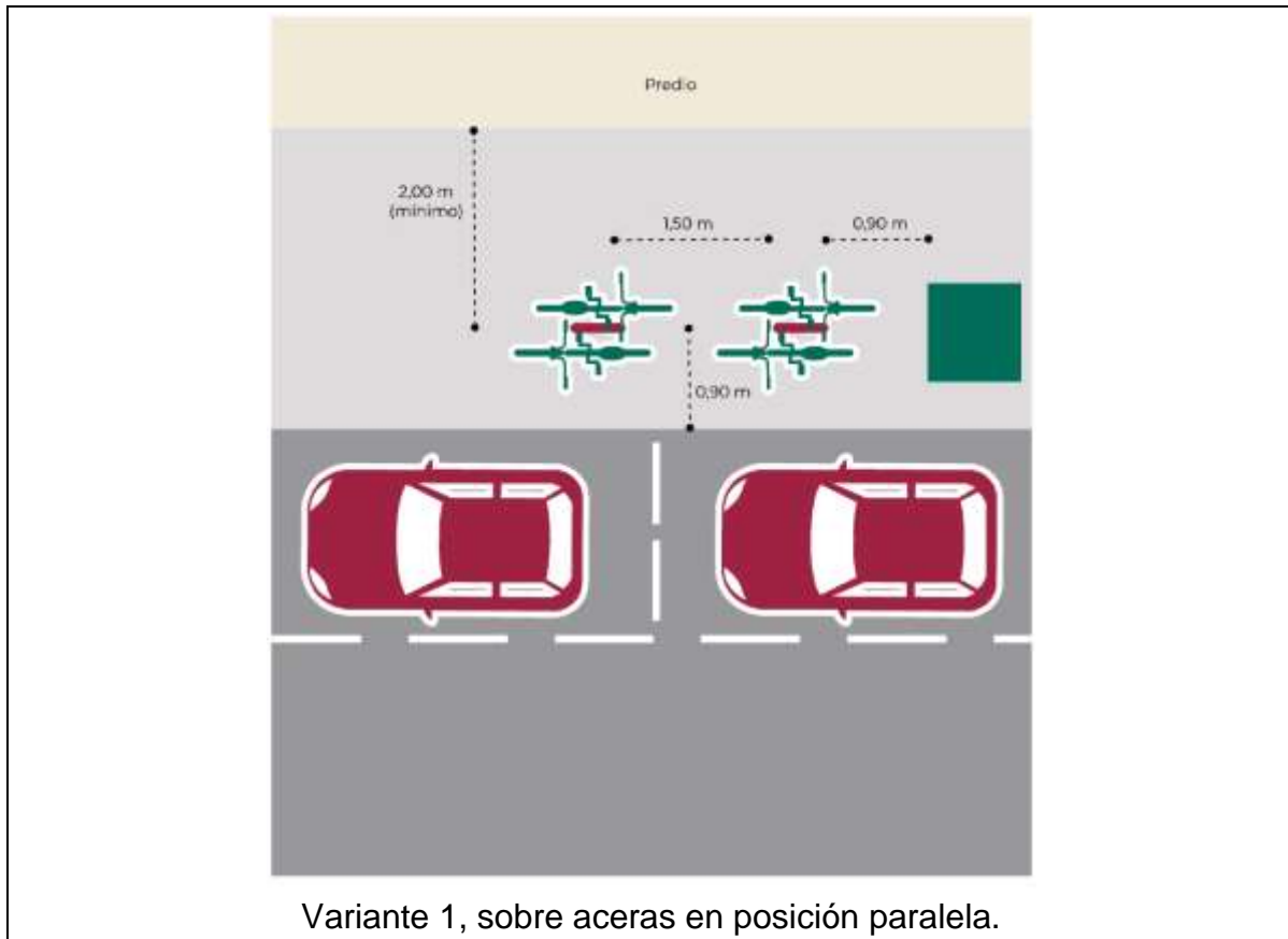
Figura 73.- Tipos de emplazamientos de biciestacionamientos en la calle [1] [2]
