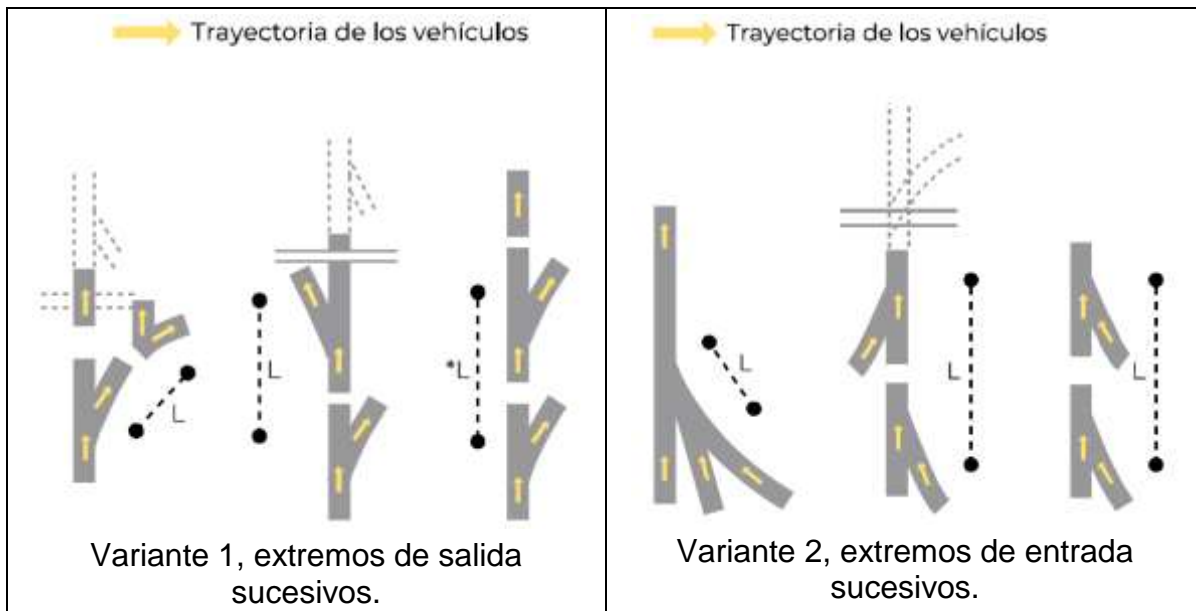
Figura 93.- Distancia entre extremos de ramales sucesivos [1] [2]
