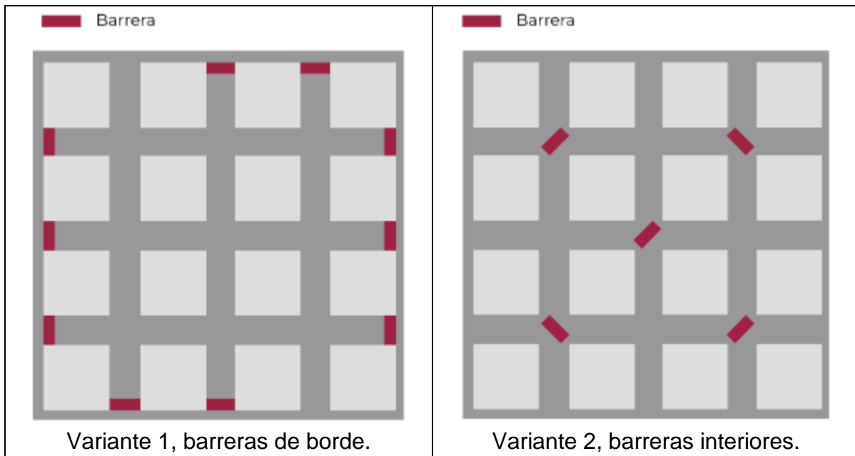
Figura 96.- Esquemas de ordenación para la moderación de tránsito en áreas delimitadas [1] [2]
