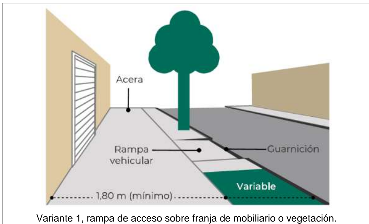
Figura 39.- Configuración de circulación peatonal con acceso vehicular [1] [2]
