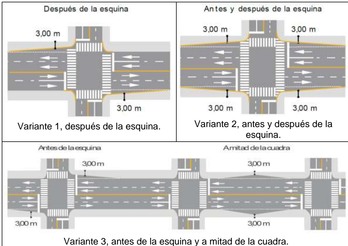
Figura 79.- Diseño mínimo para paradas de autobuses (áreas de transferencia) [1] [2]
