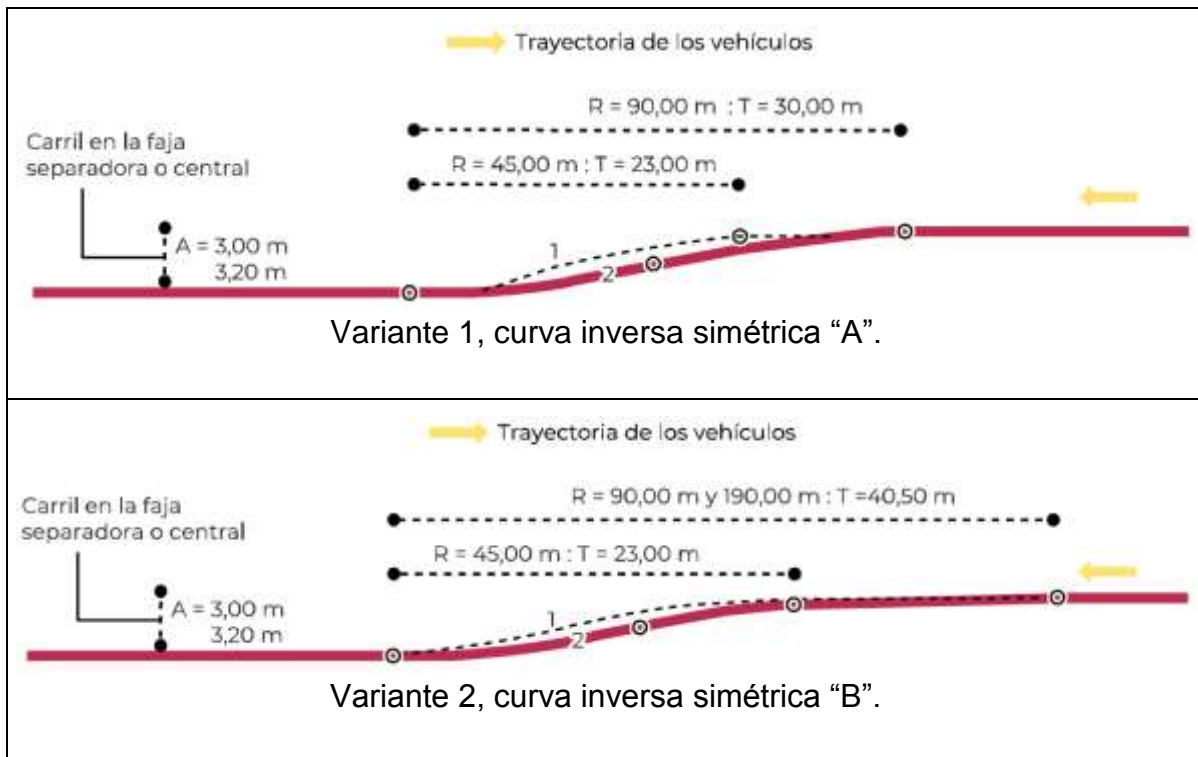
Figura 83.- Transición del carril en la faja separadora central [1] [2]
