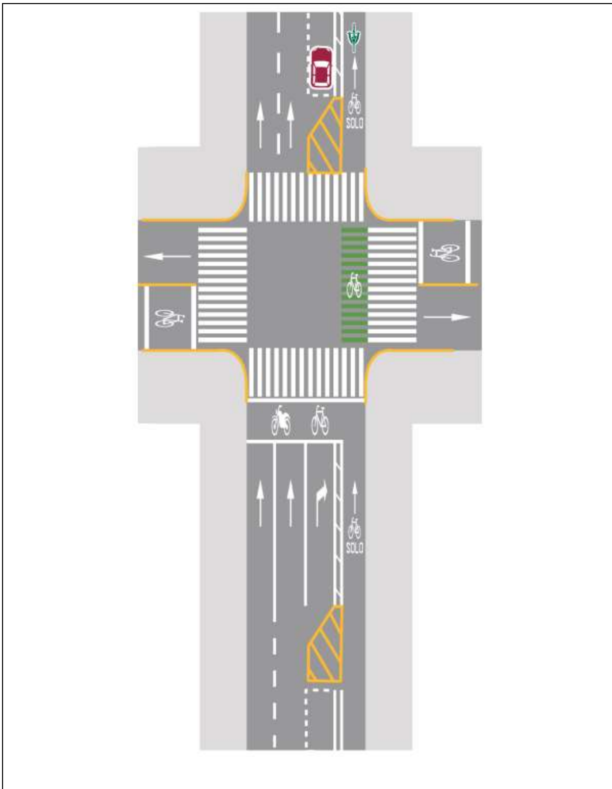
Figura 54.- Configuración de carriles para vuelta derecha en ciclovías unidireccionales confinadas por cordón de estacionamiento [1] [2]
