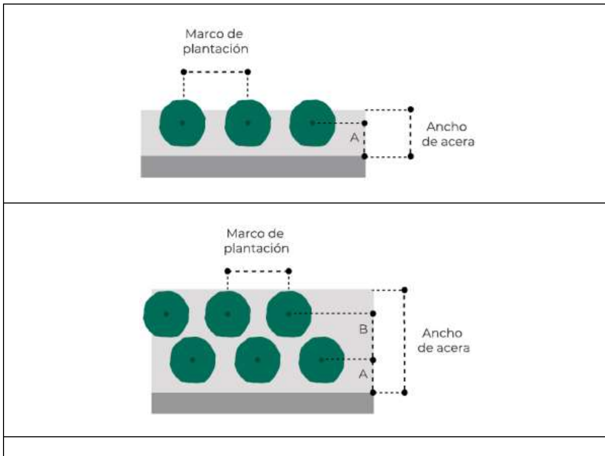
Figura 110.- Dimensiones de referencia para la colocación de árboles en las banquetas. [1] [2]
