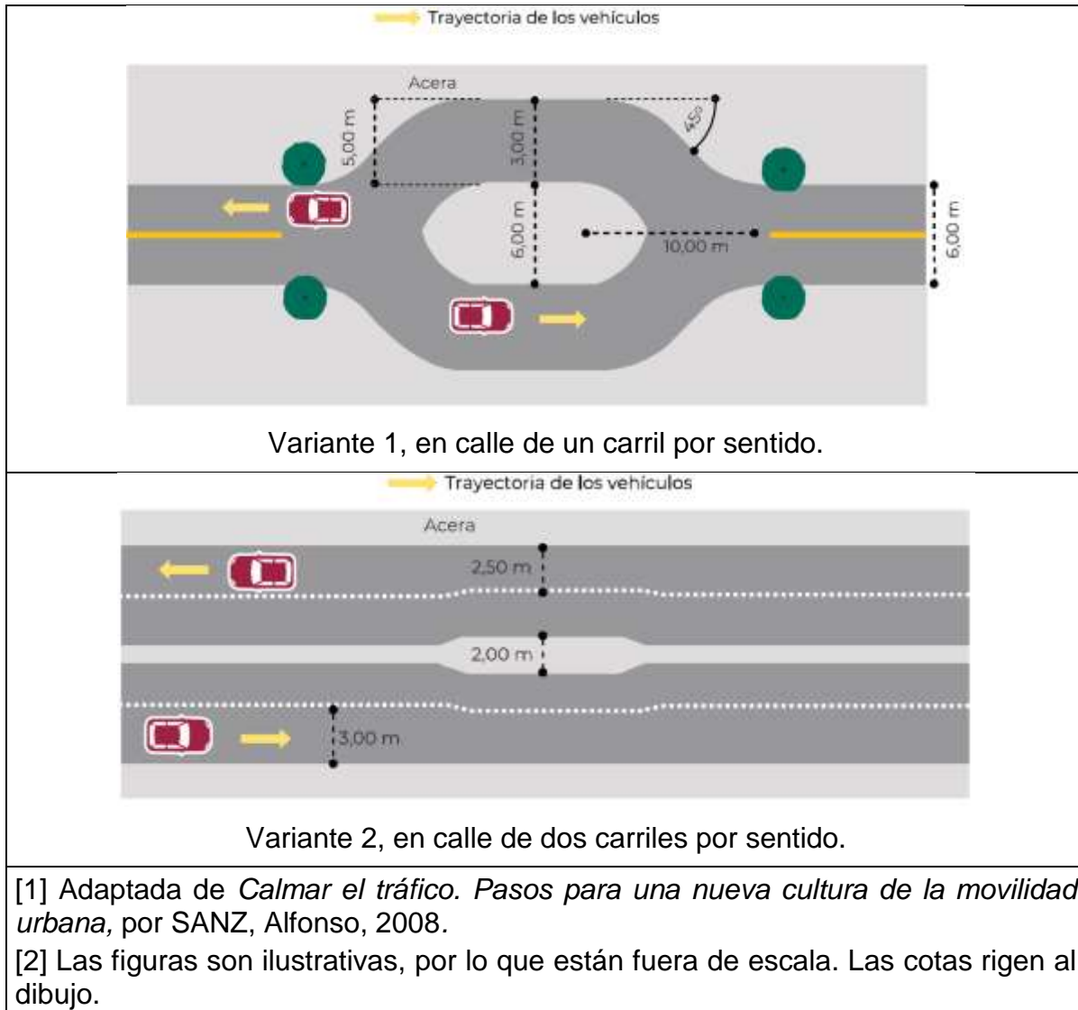
Figura 108.- Tipos de estrechamiento central [1] [2]
