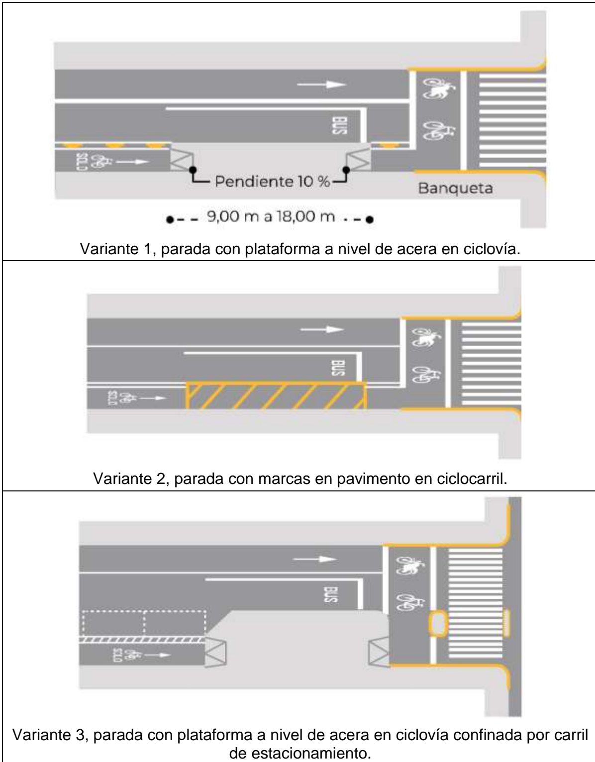
Figura 61.- Tratamientos de paradas de transporte público [1] [2]
