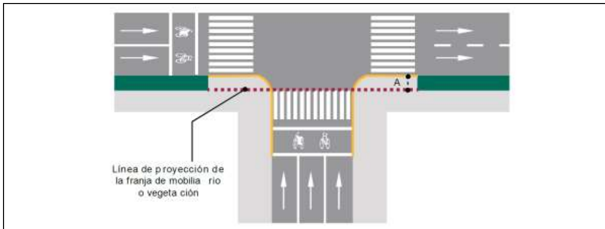
Figura 43.- Cruce peatonal remetido con respecto a la franja de mobiliario o vegetación [1] [2]
