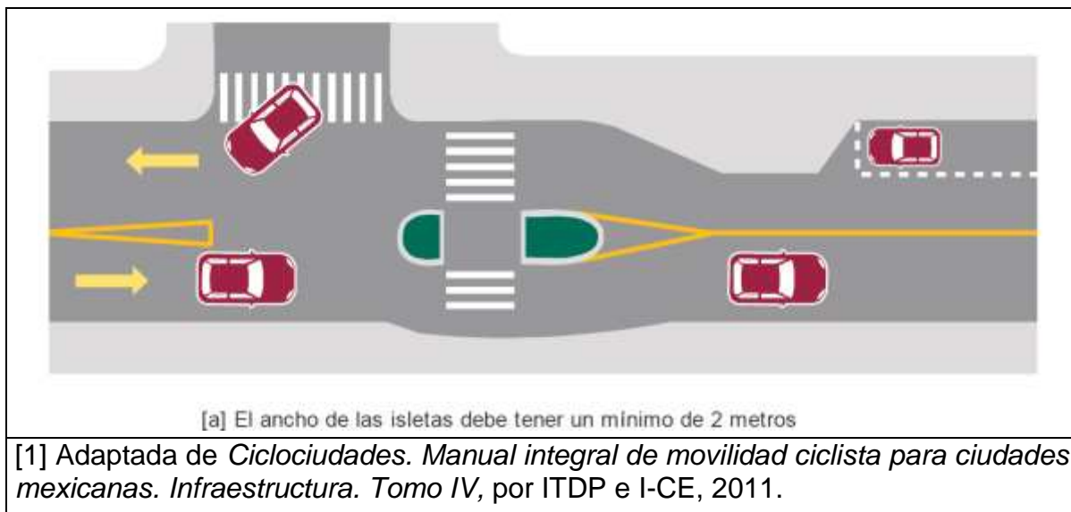
Figura 100.- Isleta [1] [2] [a]
