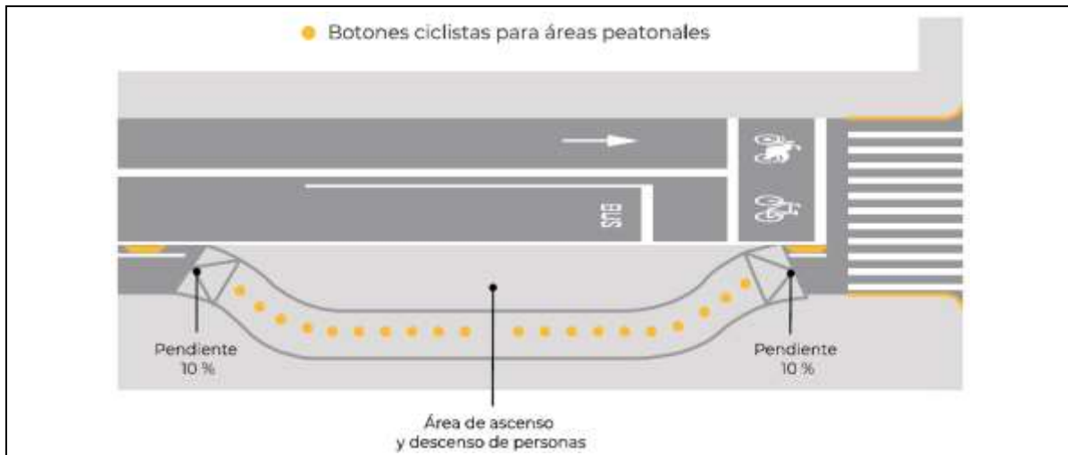
Figura 62.- Parada de transporte público con desvío ciclista [1] [2]
