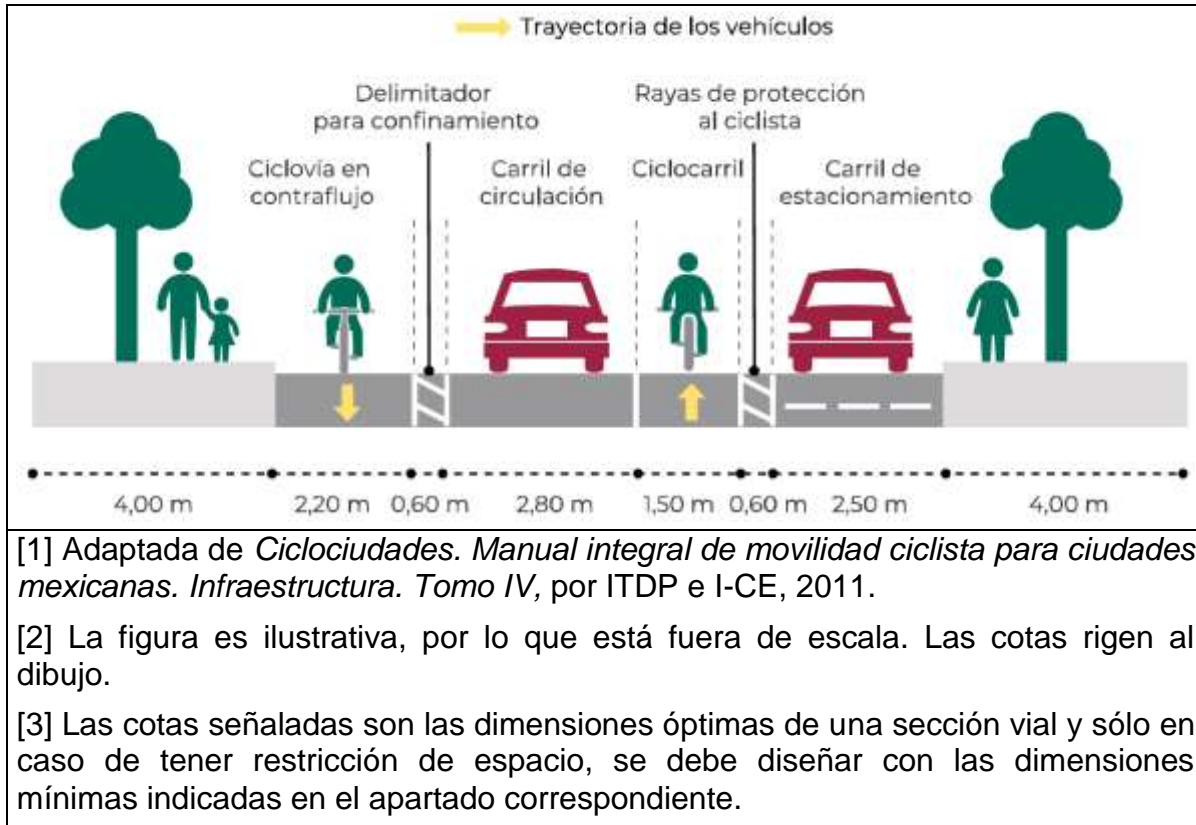
Figura 59.- Perfil tipo de vías ciclistas en contraflujo [1] [2] [3]
