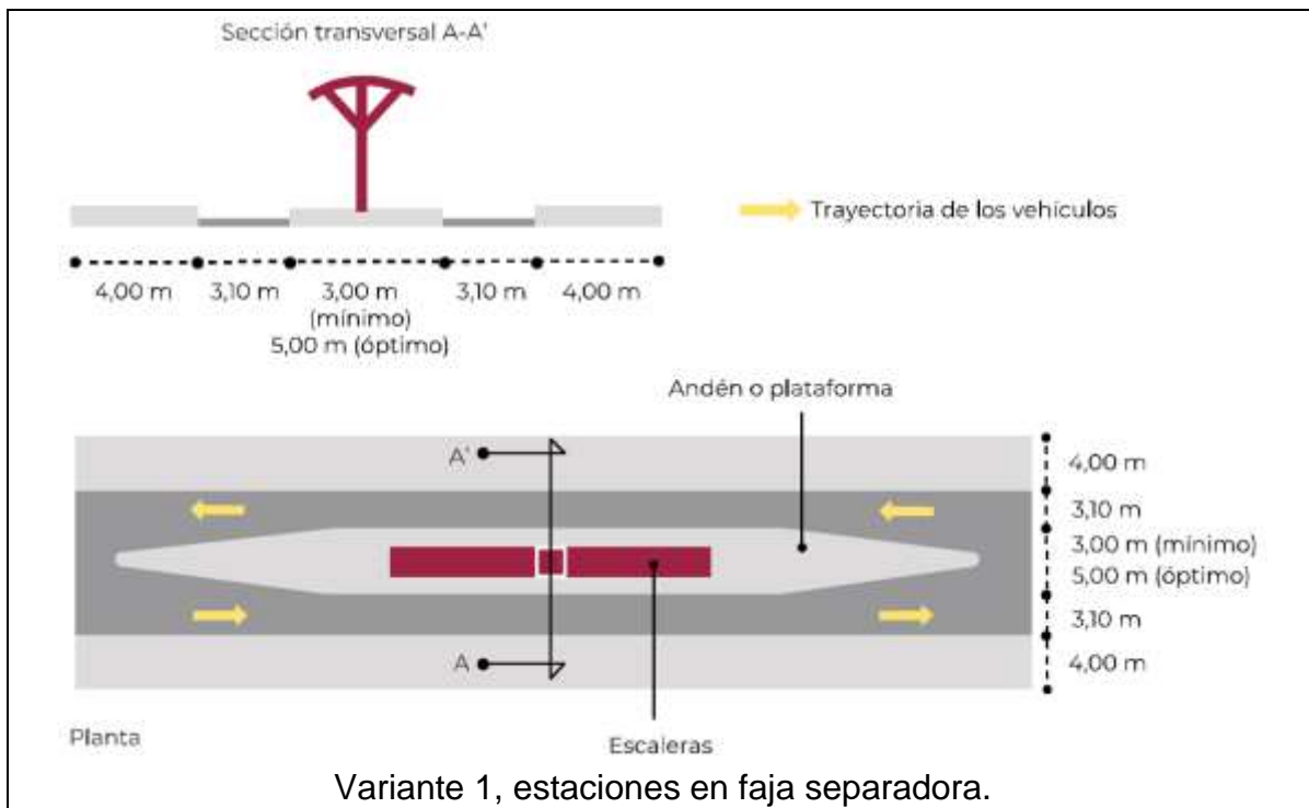
Figura 80.- Estaciones en vías exclusivas para el transporte público de pasajeros [1] [2]
