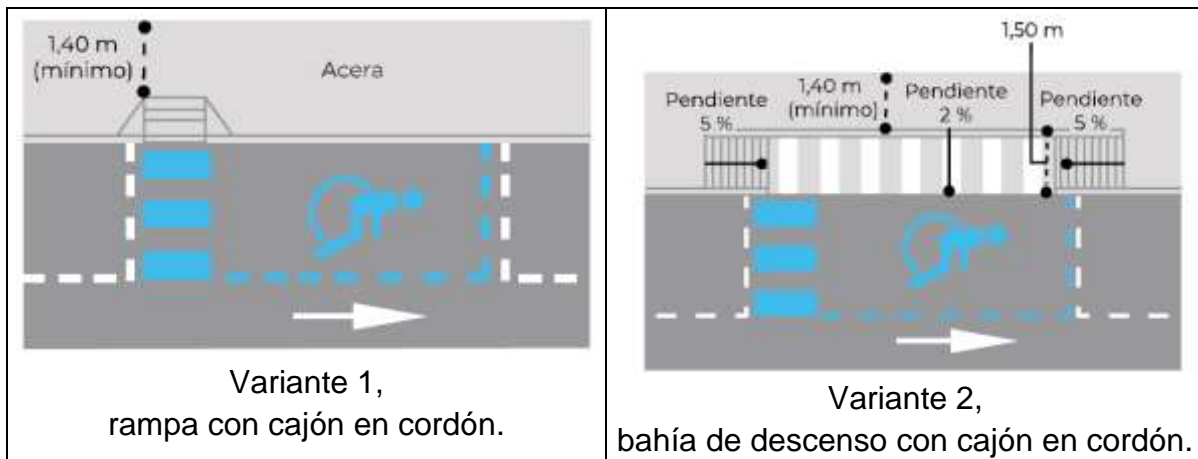
Figura 75.- Disposición de las rampas y franjas de circulación en los cajones para vehículos de personas con discapacidad [1] [2]
