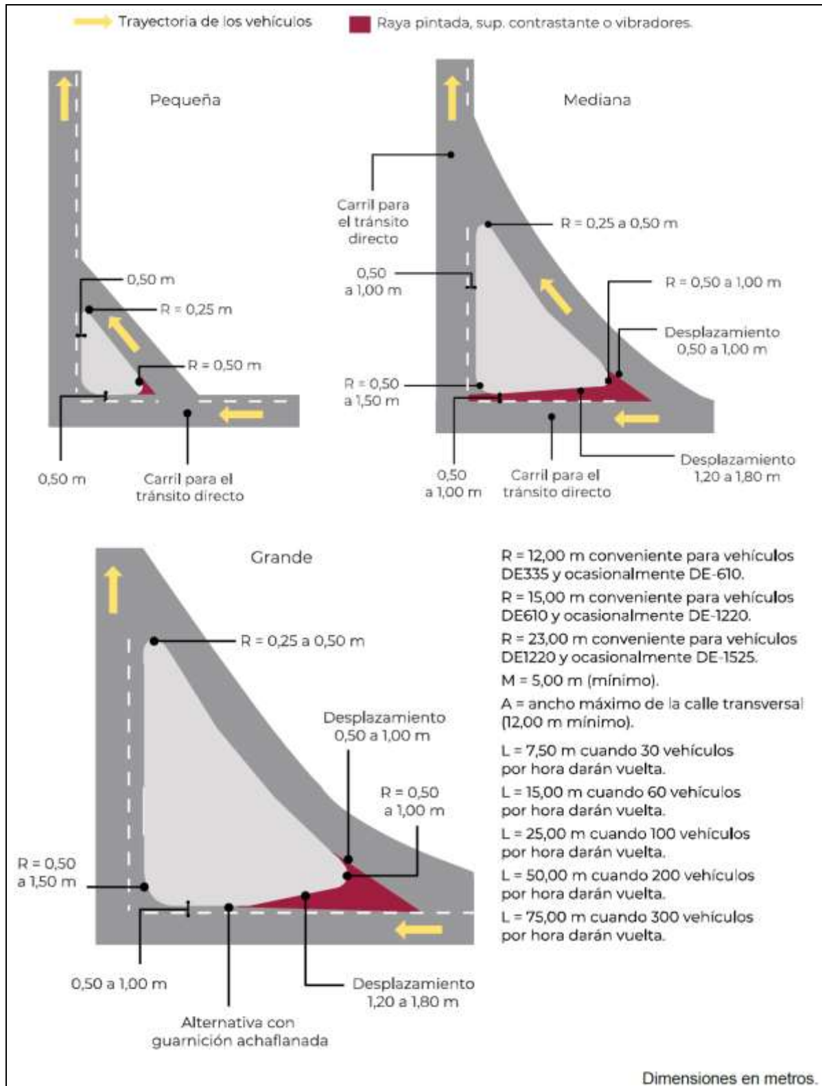
Figura 86.- Diseño de islas en intersecciones [1] [2]
