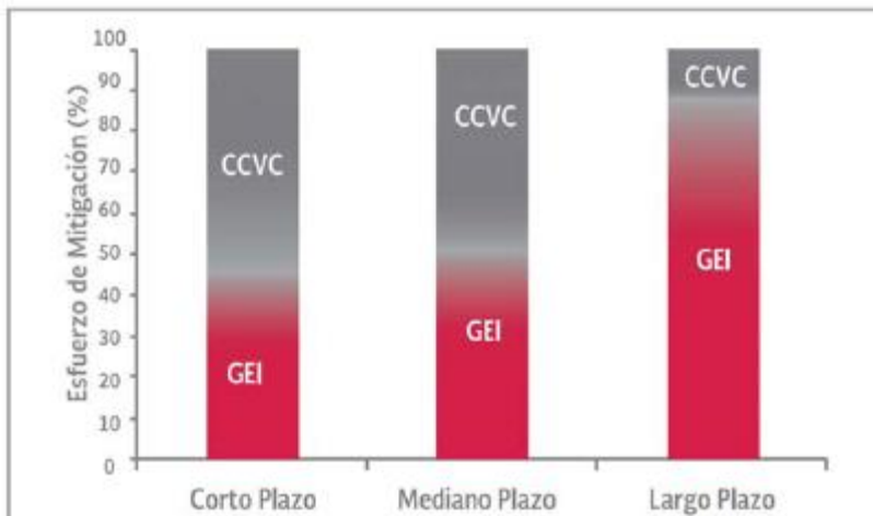
Figura 14. Representación conceptual de la participación de GEI y CCVC en los esfuerzos de mitigación.
