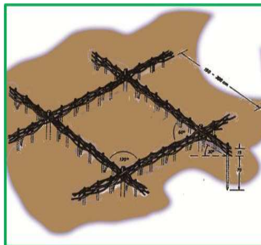
Fig. 40. Colocación en diagonal de empalizadas trenzadas.
